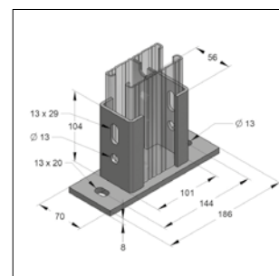
Houter voor dubbele montagerail C-profiel 45/90
