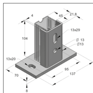
Houter 45 haaks voor montagerail
